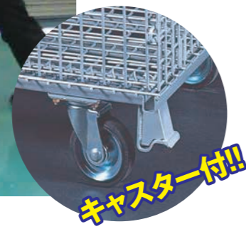
写真はSC-3S 150φゴムキャスター(固定2輪、自在2輪、ストッパー付)
